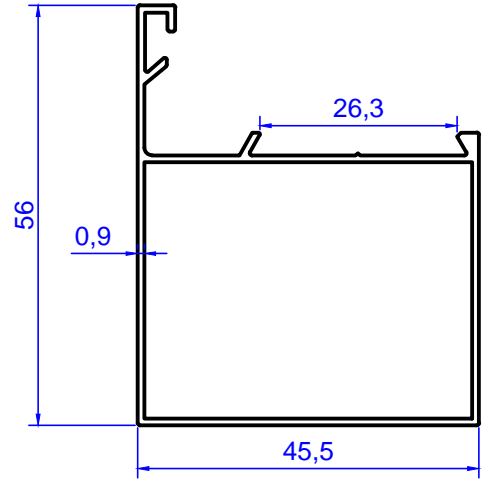
Profil No: 2130 Gramaj : 0,497 kg/m
