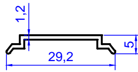
Profil No: 2054 Gramaj : 0,112 kg/m
