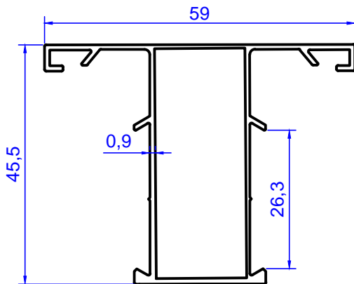
Profil No: 2128 Gramaj : 0,522 kg/m
