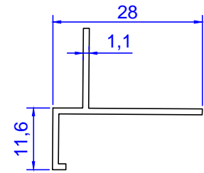
Profil No: 2500 Gramaj : 0,164 kg/m
