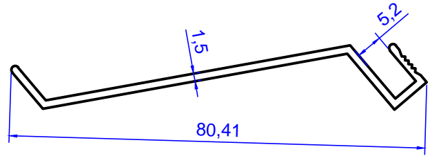
Profil No: 3017 Gramaj : 0,398 kg/m
