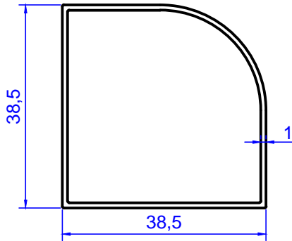
Profil No: 2135 Gramaj : 0,384 kg/m
