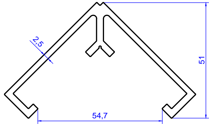
Profil No: 2118 Gramaj : 1,275 kg/m
