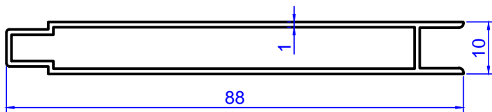
Profil No: 2077 Gramaj : 0,524 kg/m
