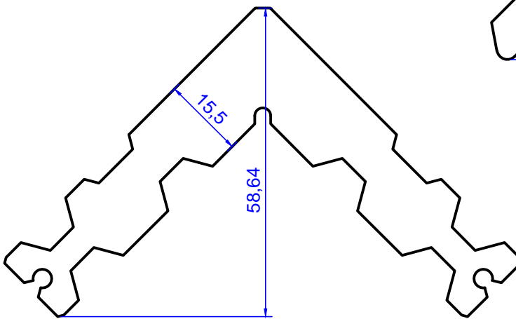
Profil No: 2036 Gramaj : 4,245 kg/m
