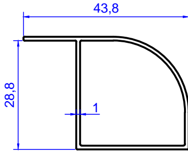
Profil No: 2133 Gramaj : 0,327 kg/m
