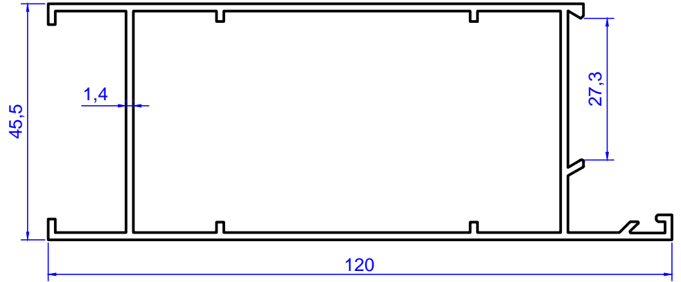
Profil No: 2090 Gramaj : 1,266 kg/m
