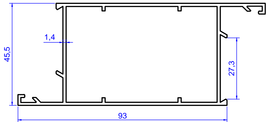
Profil No: 2092 Gramaj : 1,149 kg/m
