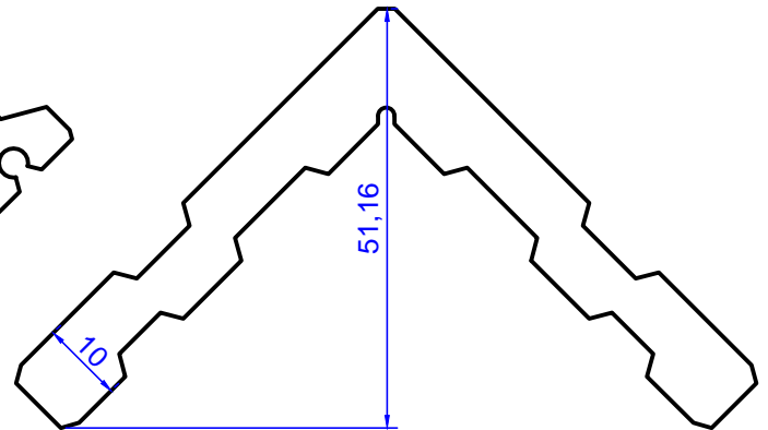
Profil No: 2037 Gramaj : 2,787 kg/m
