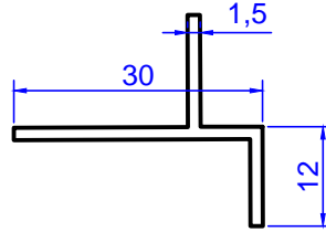
Profil No: 3014 Gramaj : 0,220 kg/m
