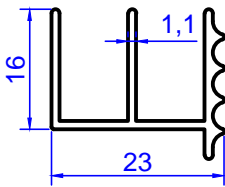
Profil No: 2112 Gramaj : 0,231 kg/m
