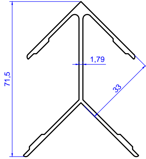
Profil No: 2119 Gramaj : 0,937 kg/m
