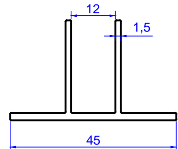
Profil No: 3189 Gramaj : 0,447 kg/m
