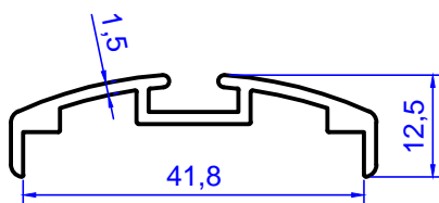
Profil No: 2011 Gramaj : 0,341 kg/m
