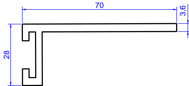
Profil No: 2042 Gramaj : 0,251 kg/m
