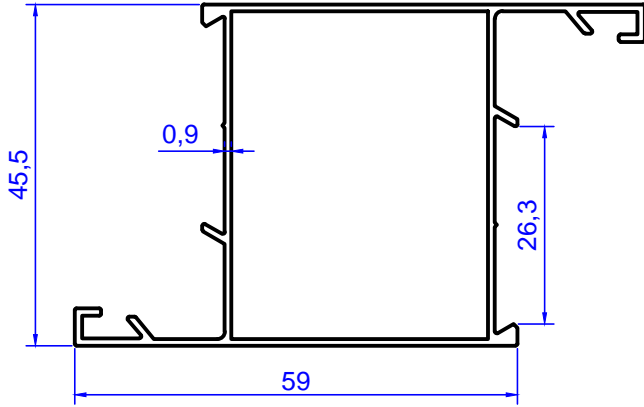
Profil No: 2132 Gramaj : 0,605 kg/m
