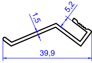
Profil No: 3016 Gramaj : 0,218 kg/m
