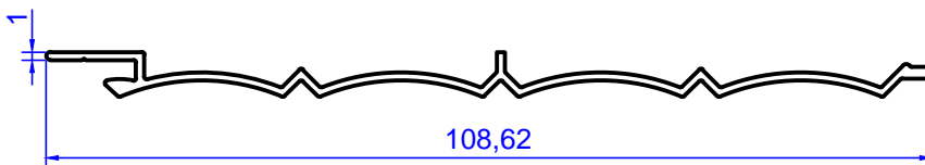
Profil No: 2111 Gramaj : 0,354 kg/m
