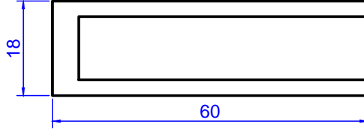
Profil No: 2016 Gramaj : 1,138 kg/m
