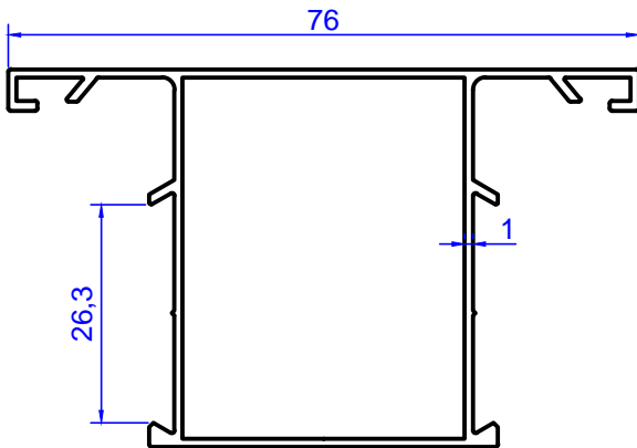
Profil No: 2081 Gramaj : 0,663 kg/m
