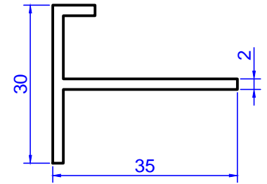
Profil No: 2041 Gramaj : 0,374 kg/m
