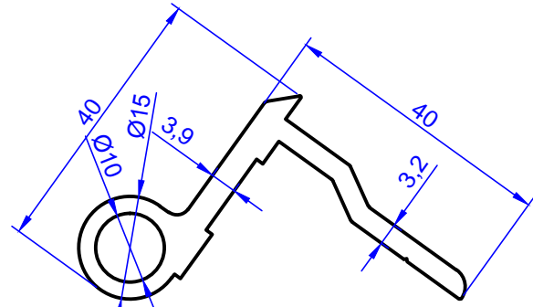
Profil No: 2089 Gramaj : 0,894 kg/m
