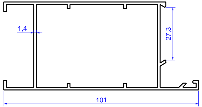
Profil No: 2093 Gramaj : 1,130 kg/m
