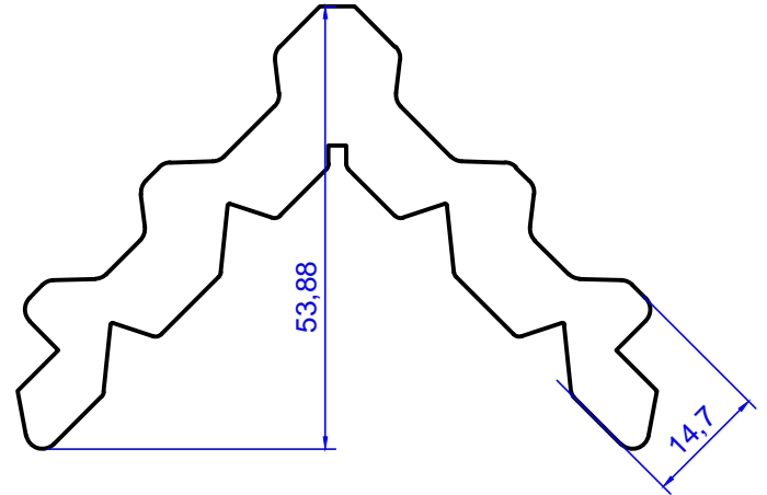
Profil No: 2032 Gramaj : 3,170 kg/m
