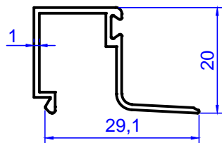
Profil No: 2097 Gramaj : 0,211 kg/m
