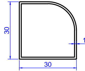
Profil No: 2121 Gramaj : 0,297 kg/m
