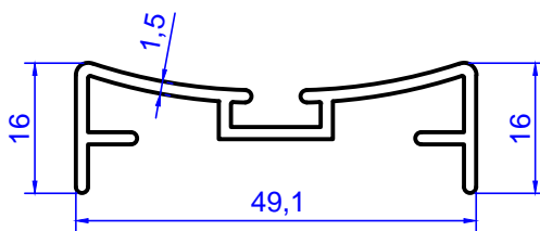
Profil No: 3141 Gramaj : 0,421 kg/m
