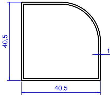
Profil No: 2122 Gramaj : 0,405 kg/m
