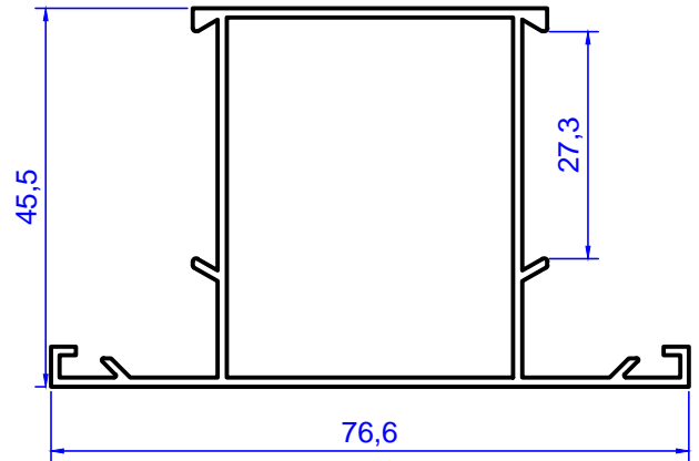
Profil No: 2095 Gramaj : 0,702 kg/m
