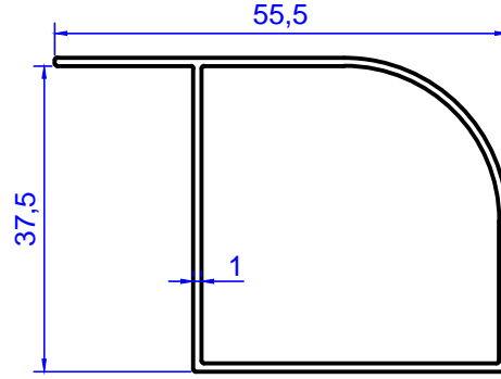
Profil No: 2134 Gramaj : 0,430 kg/m
