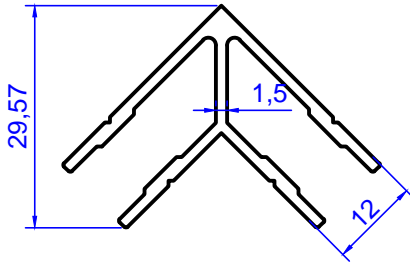
Profil No: 2057 Gramaj : 0,481 kg/m
