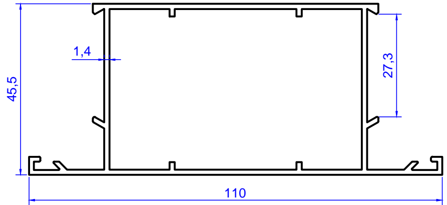
Profil No: 2091 Gramaj : 1,149 kg/m
