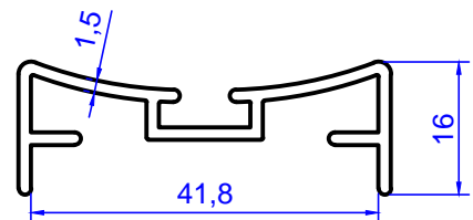
Profil No: 2012 Gramaj : 0,404 kg/m
