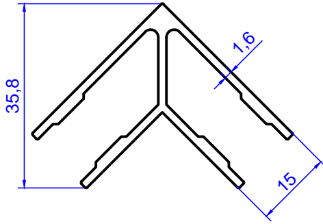
Profil No: 4489 Gramaj : 0,640 kg/m
