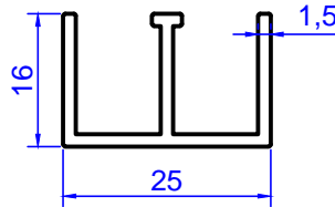
Profil No: 3022 Gramaj : 0,287 kg/m
