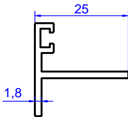
Profil No: 2055 Gramaj : 0,262 kg/m
