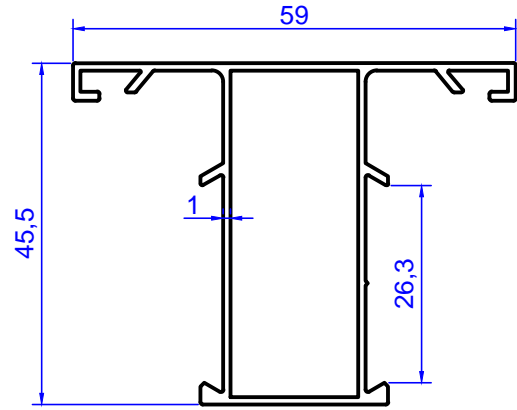
Profil No: 2078 Gramaj : 0,572 kg/m
