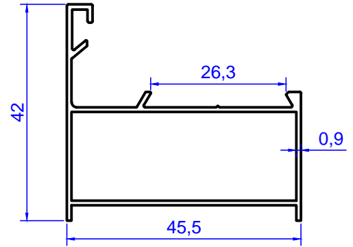
Profil No: 2127 Gramaj : 0,429 kg/m
