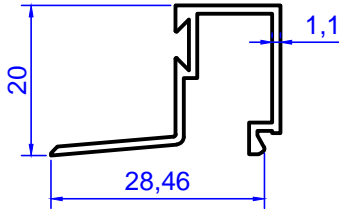
Profil No: 2017 Gramaj : 0,229 kg/m
