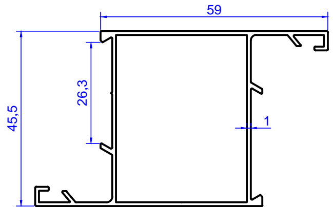
Profil No: 2082 Gramaj : 0,657 kg/m
