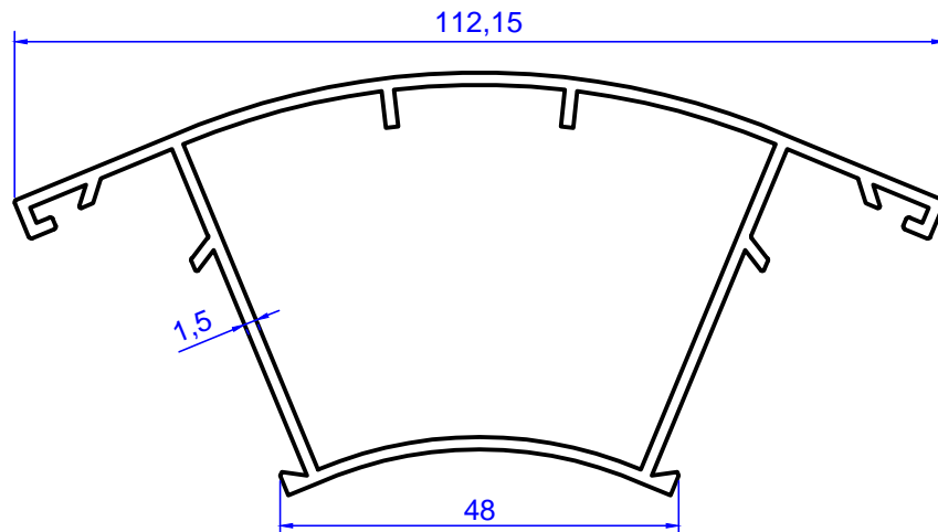
Profil No: 3091 Gramaj : 1,163 kg/m
