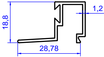
Profil No: 2018 Gramaj : 0,244 kg/m
