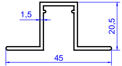
Profil No: 3010 Gramaj : 0,341 kg/m
