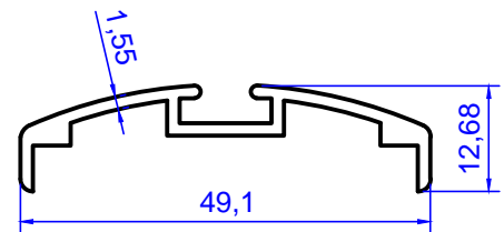
Profil No: 3142 Gramaj : 0,355 kg/m
