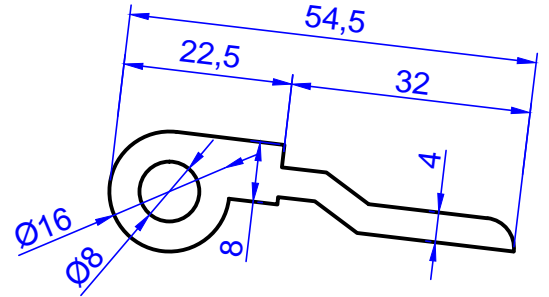
Profil No: 2014 Gramaj : 0,934 kg/m
