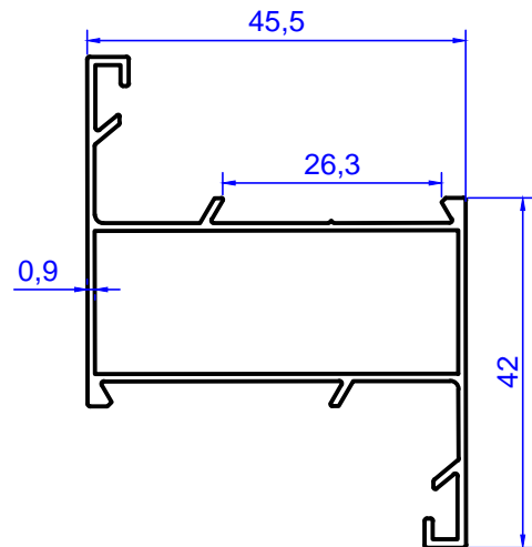
Profil No: 2129 Gramaj : 0,522 kg/m
