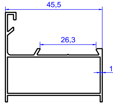
Profil No: 2080 Gramaj : 0,472 kg/m
