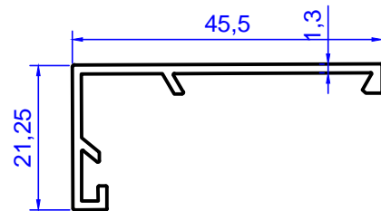
Profil No: 2070 Gramaj : 0,294 kg/m
