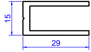
Profil No: 2068 Gramaj : 0,403 kg/m
