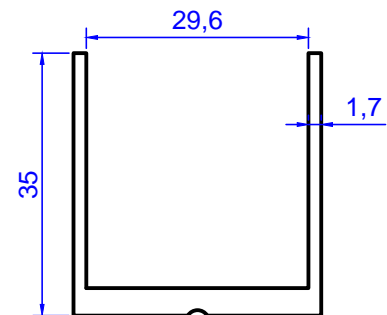
Profil No: 2120 Gramaj : 0,614 kg/m
