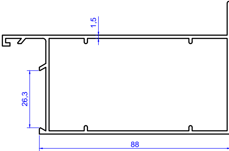
Profil No: 2071 Gramaj : 1,284 kg/m
