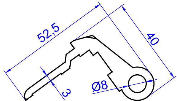
Profil No: 2066 Gramaj : 1,173 kg/m
