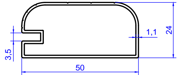
Profil No: 2123 Gramaj : 0,450 kg/m
