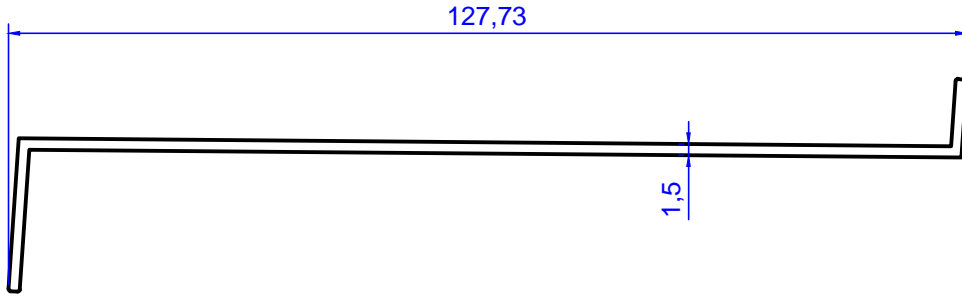
Profil No: 3225 Gramaj : 0,623 kg/m
