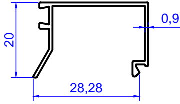
Profil No: 2126 Gramaj : 0,192 kg/m
