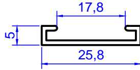
Profil No: 3012 Gramaj : 0,125 kg/m
