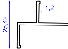
Profil No: 2059 Gramaj : 0,174 kg/m
