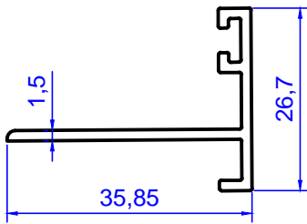
Profil No: 3079 Gramaj : 0,298 kg/m
