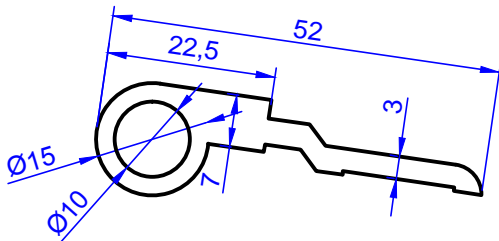
Profil No: 2065 Gramaj : 0,696 kg/m
