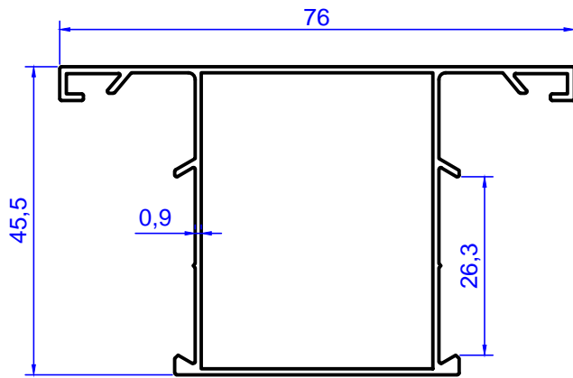
Profil No: 2131 Gramaj : 0,605 kg/m
