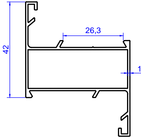
Profil No: 2079 Gramaj : 0,572 kg/m
