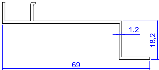
Profil No: 2053 Gramaj : 0,339 kg/m
