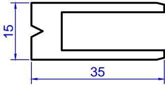
Profil No: 2015 Gramaj : 0,676 kg/m
