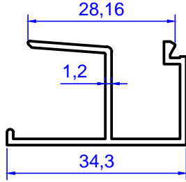
Profil No: 2073 Gramaj : 0,296 kg/m
