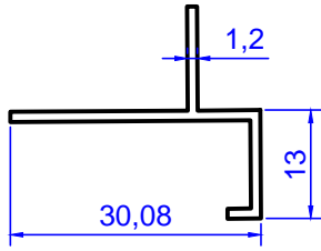
Profil No: 3013 Gramaj : 0,186 kg/m
