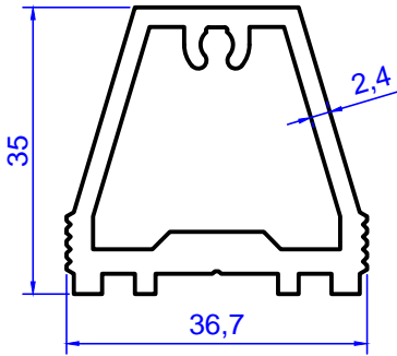
Profil No: 2117 Gramaj : 1,028 kg/m
