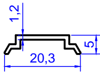
Profil No: 2052 Gramaj : 0,084 kg/m
