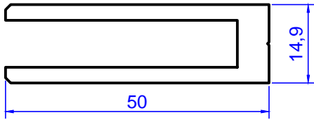
Profil No: 2033 Gramaj : 0,954 kg/m
