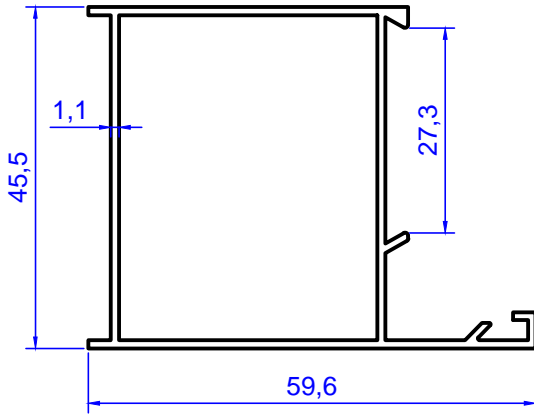
Profil No: 2094 Gramaj : 0,607 kg/m
